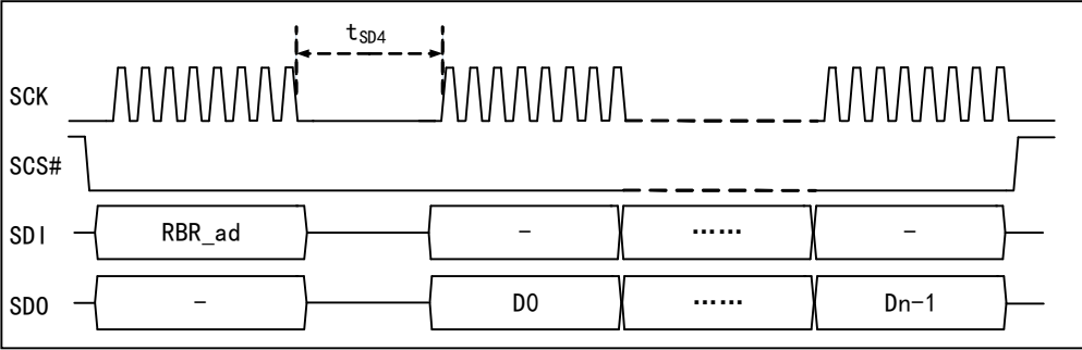
图 9-5 SPI 模式读 FIFO
