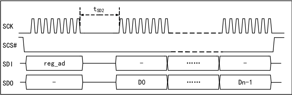
图 9-3 SPI 模式读寄存器
