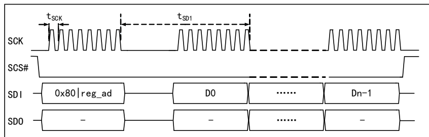
图 9-2 SPI 模式写寄存器
