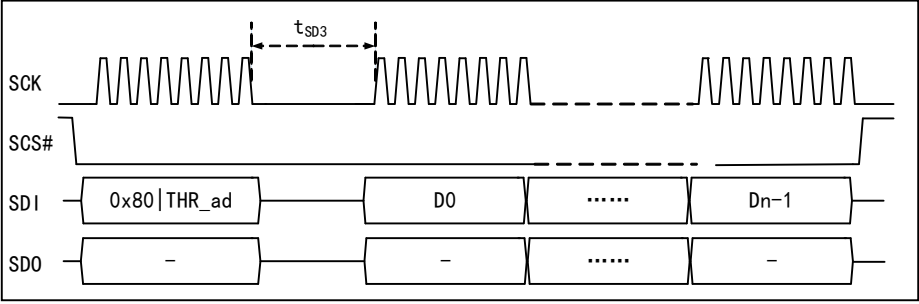
图 9-4 SPI 模式写 FIFO
