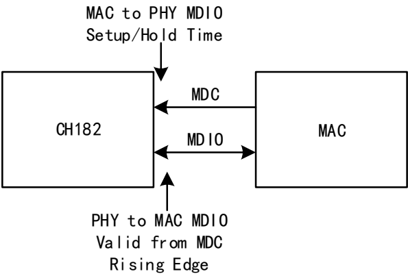
图 7-8 MDC/MDIO 时序
