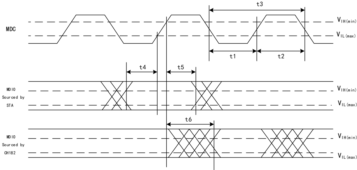
图 7-8 MDC/MDIO 时序
