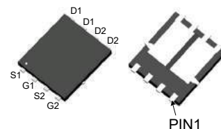
PDFN3x3
