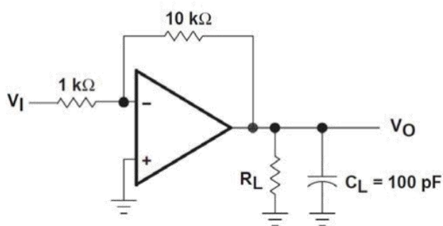
图 2. 10 倍增益电路
