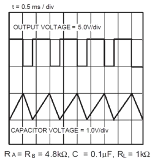
图 6 非稳态波形图
