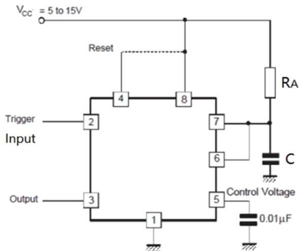
图 3 单稳态电路
