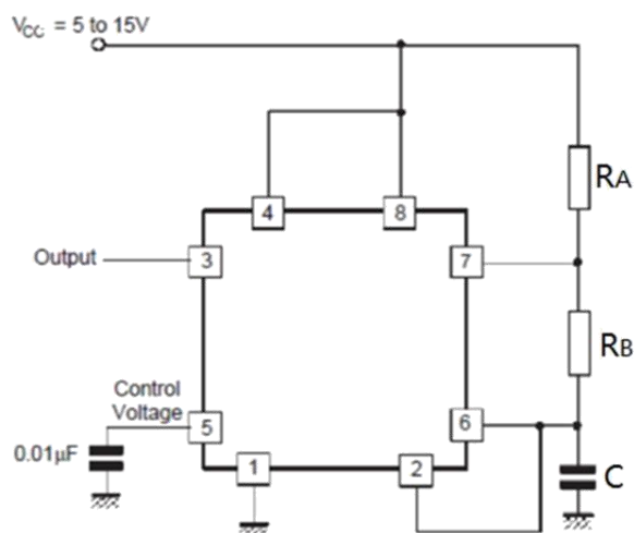
图 5 非稳态电路
