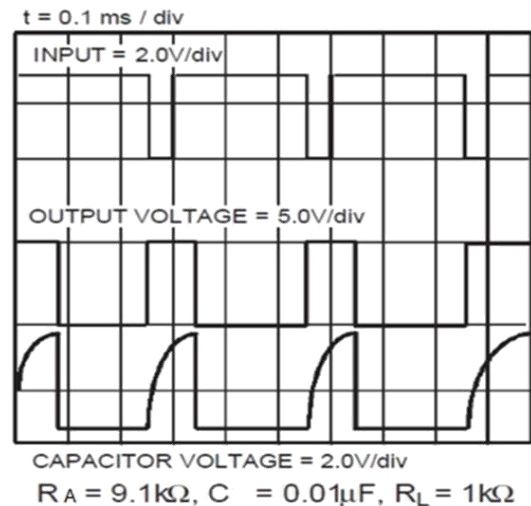
图 4 单稳态波形图
