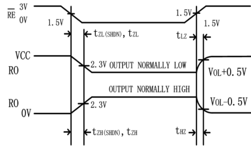
图 8 接收器使能/关断时序
