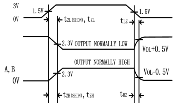
图 6 驱动器使能/关断时序
