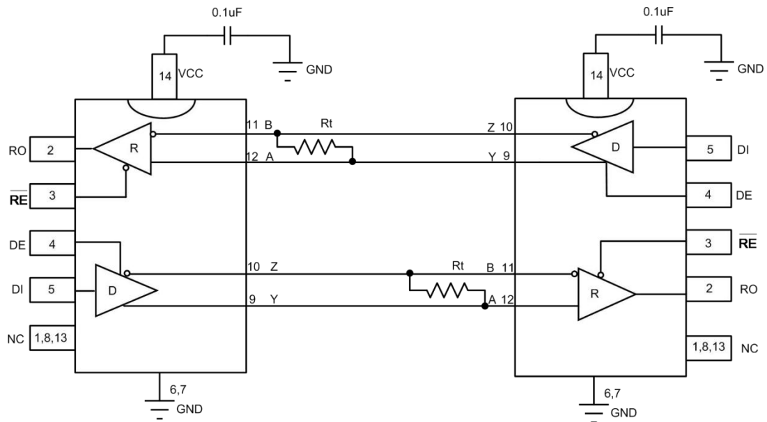
图 10 HGX3491 和 RS-485 典型全双工工作电路
