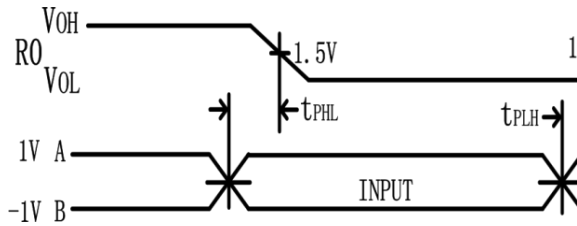
图 7 接收器传输延时
