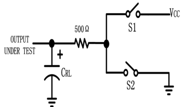
图 2 接收器使能/关断 开关特性测试负载
