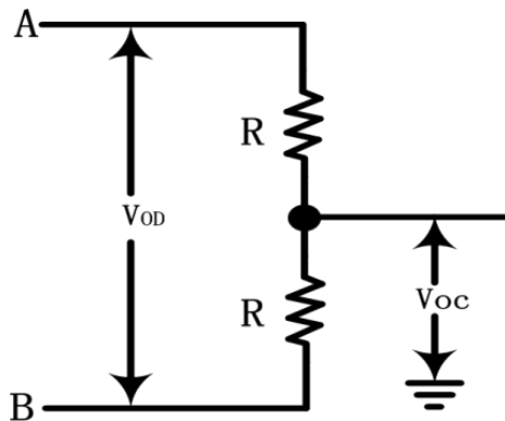
图1 驱动器直流特性测试负载
