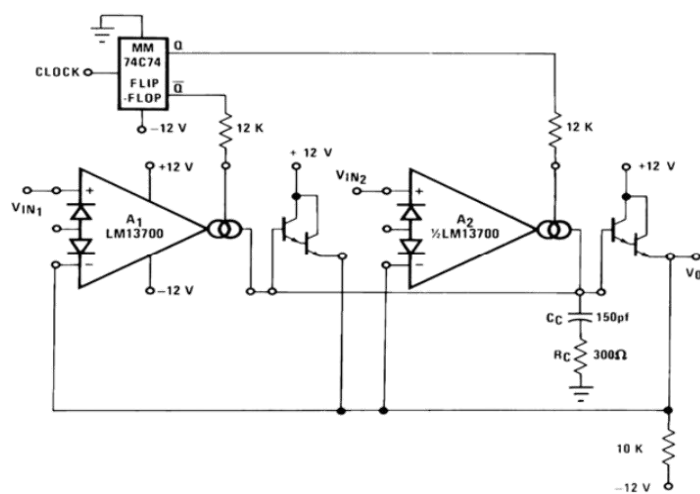
图 19 多路复用器
