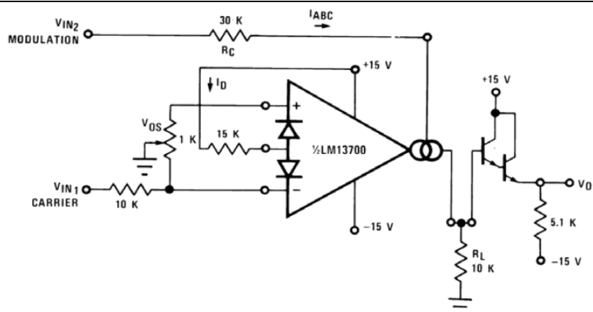
图 14 振幅调制器
