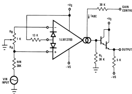
图 10 压空放大器
