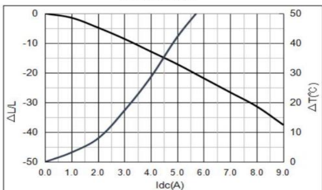
YSPI0520-2R2M
