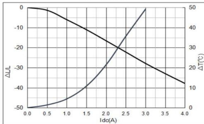
YSPI0520-100M
