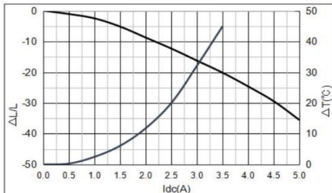
YSPI0520-100M
