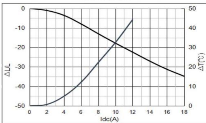
YSPI0520-1R0M
