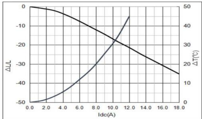
YSPI0520-R68M
