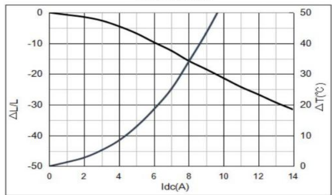
YSPI0520-1R5M
