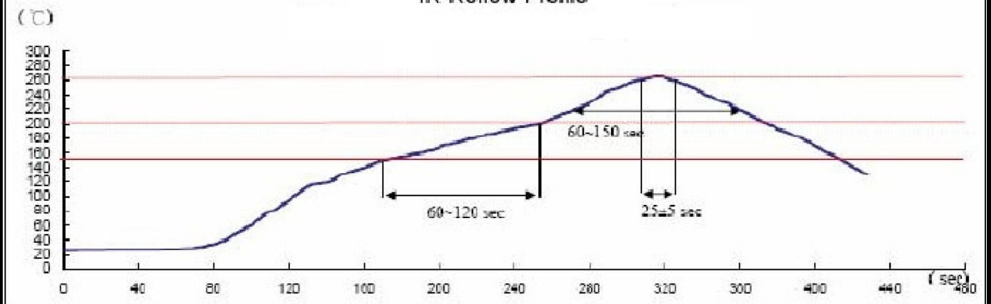
IR-Reflow Profile
