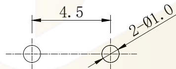
PCB线路板安装图(±0.1)
