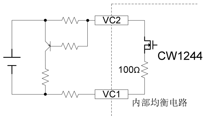
均衡功能示意图
