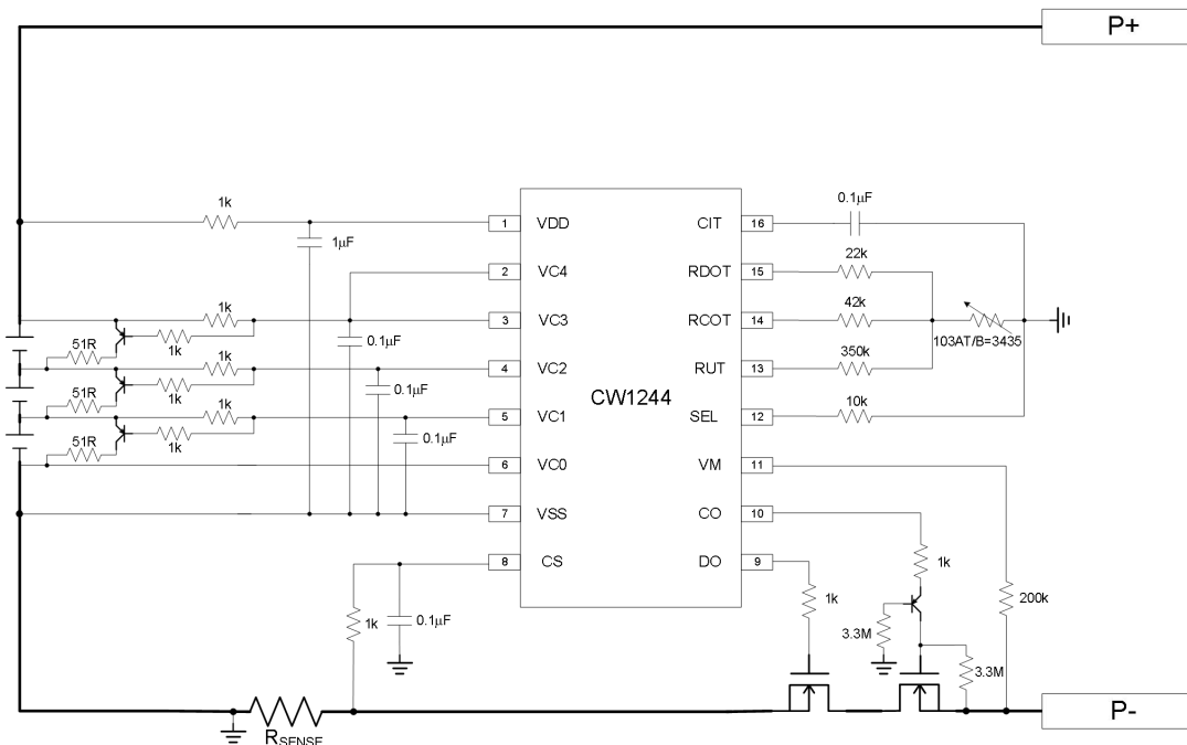
3串带均衡功能应用电路
