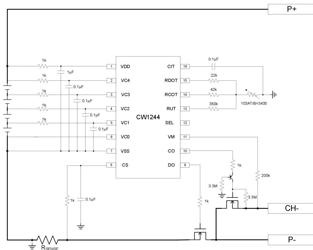
4 串异口应用电路 (CH-)
