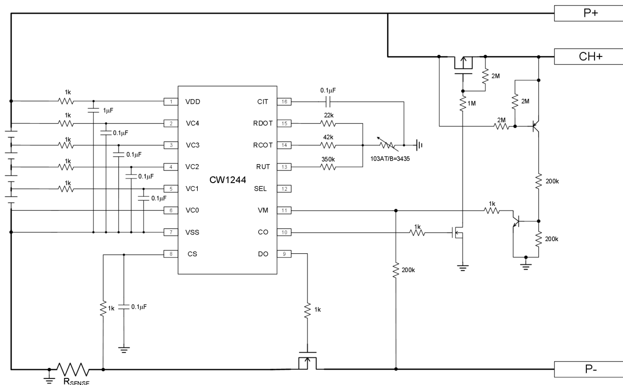
4 串异口应用电路 (CH+)
