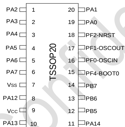
图 3-13 TSSOP20 Pinout2 PY32F030F2xPx / PY32F030F2xPx-E (Top view)
