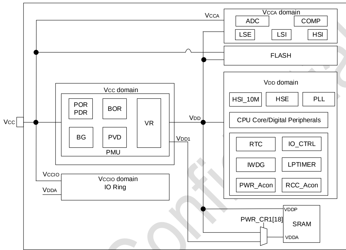
图 2-2 电源框图
