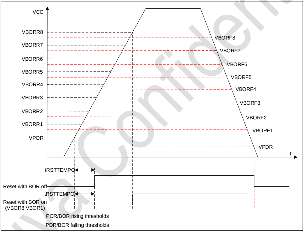
图 2-3 POR/PDR/BOR 阈值
