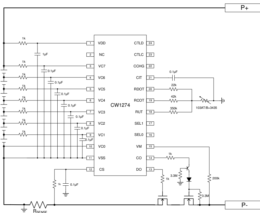
7 串不带均衡功能应用电路
