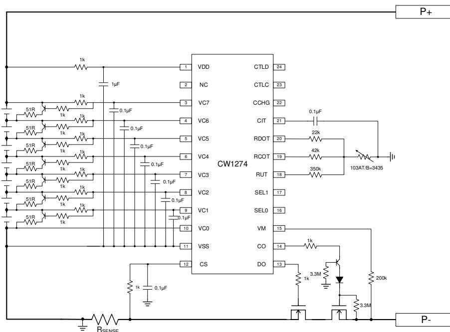
7 串带均衡功能应用电路
