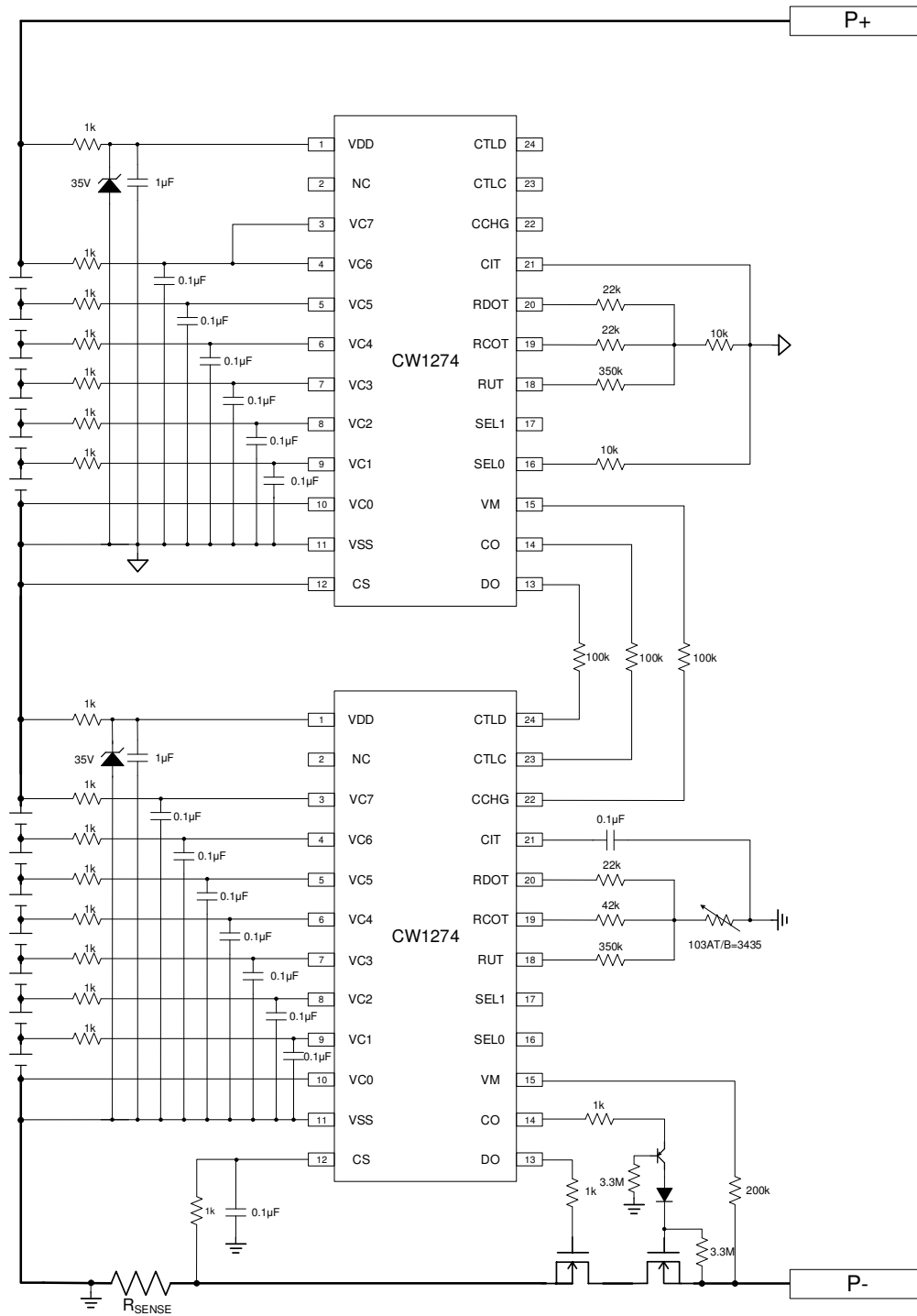
13 串不带均衡功能应用电路
