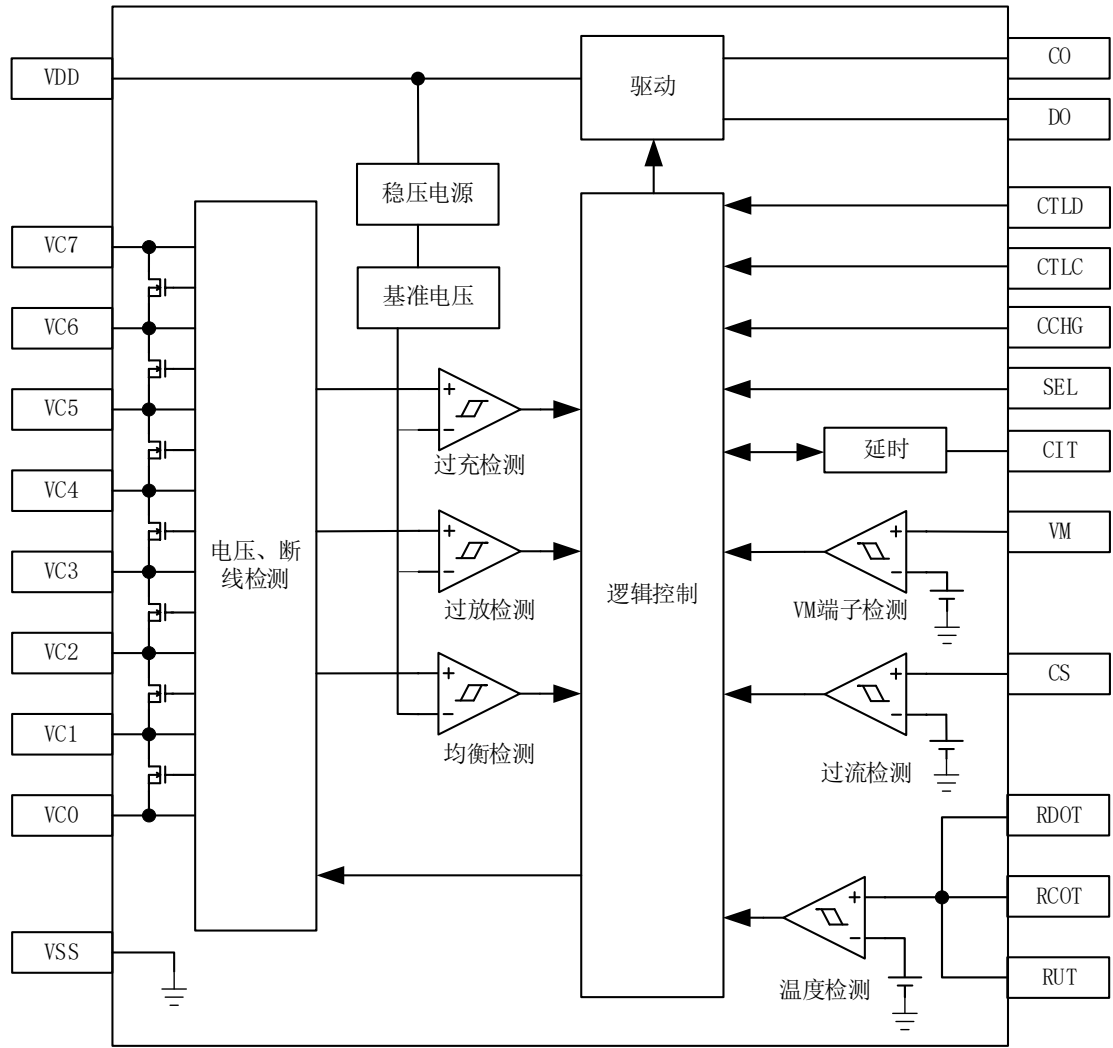
原理框图
