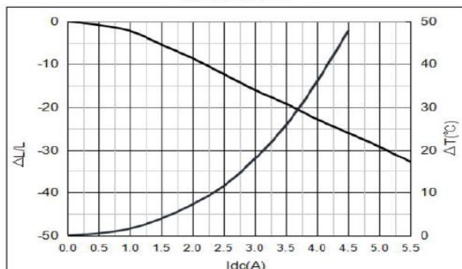
YSPI0420-2R2M
