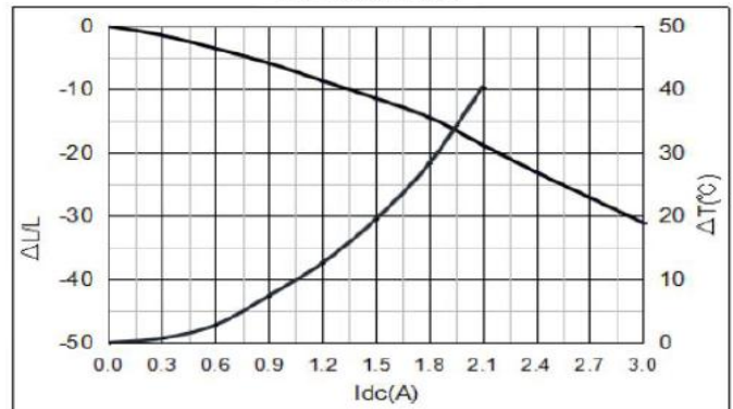
YSPI0420-8R2M
