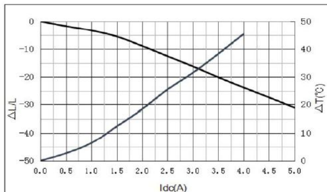
YSPI0530-8R2M
