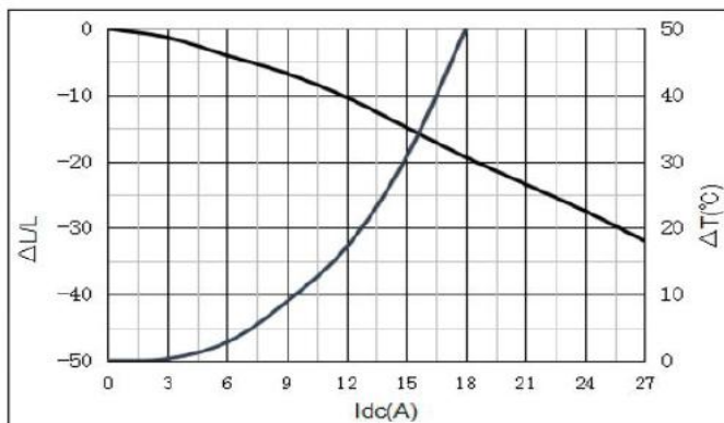
YSPI0530-R47M
