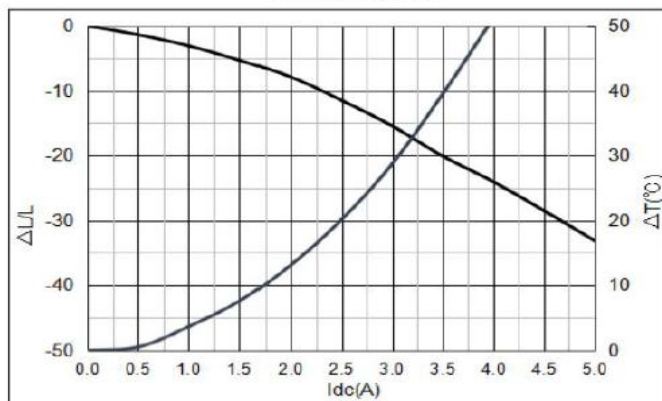
YSPI0530-8R2M
