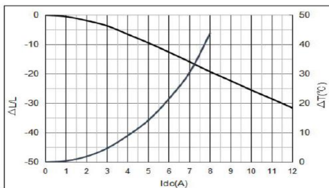
YSPI0530-1R0M
