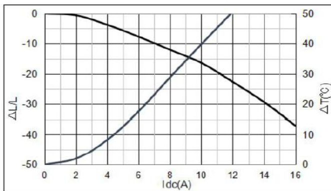
YSPI0530-R68M
