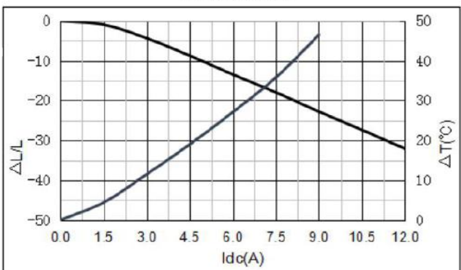
YSPI0530-1R2M
