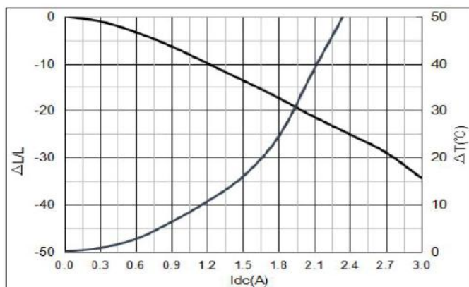
YSPI0530-220M
