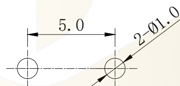
PCB线路板安装图(±0.1)
