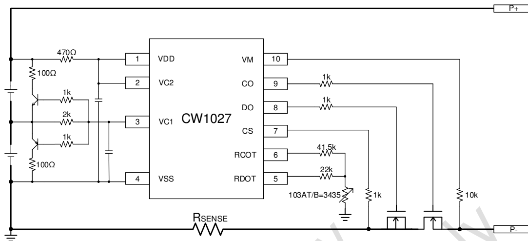
2 串带均衡功能应用电路
