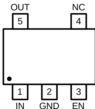
SOT23-5
