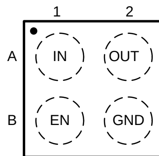
CSP-4
