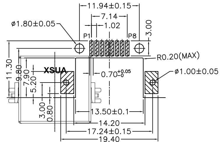
P.C.B LAYOUT
