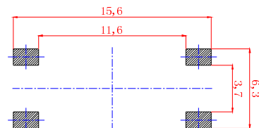
PCB. 焊接图
