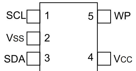
SOT-23
