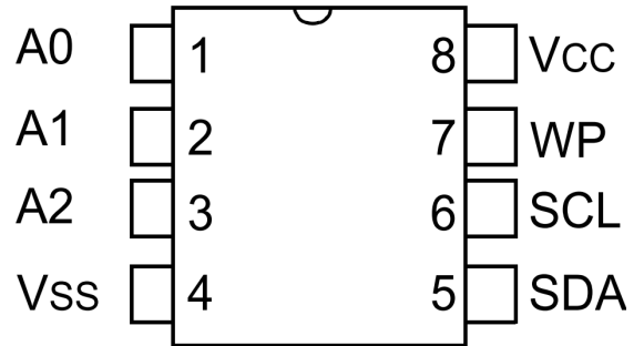
SOP8/DIP8/TSSOP8
