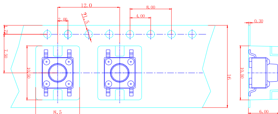
载带尺寸图
