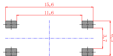
PCB. 焊接图
