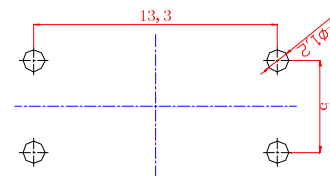
PCB. 焊接图
