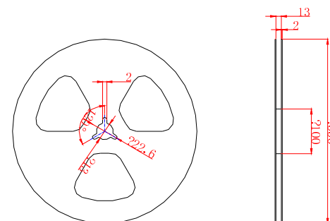
编带盘尺寸图
