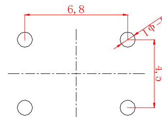
PCB参考图
