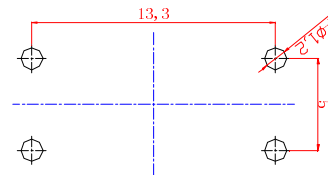
PCB. 焊接图
