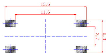
PCB. 焊接图
