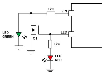
图 6 LED 双灯应用电路
