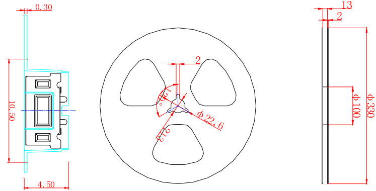
编带盘尺寸图
