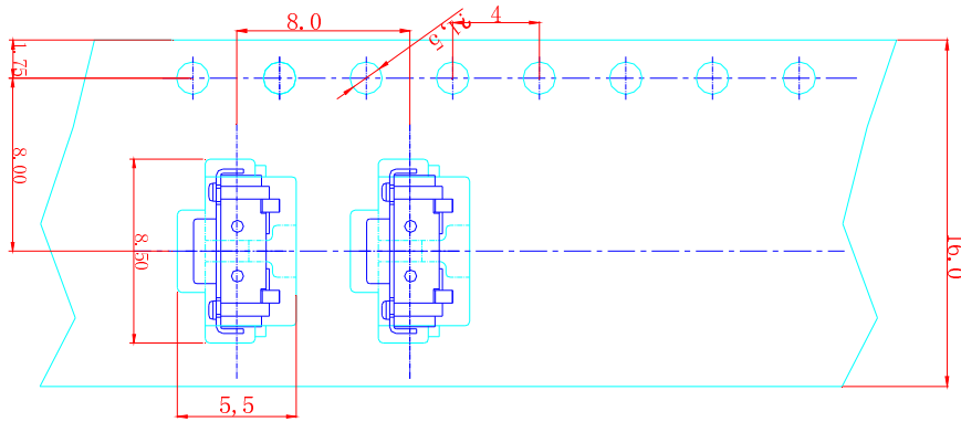
载带尺寸图
