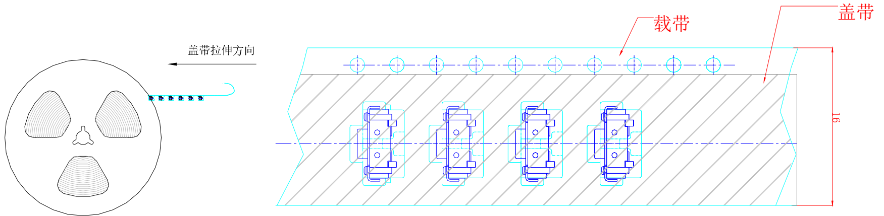
包装图
