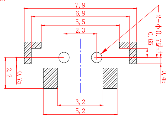
P C B 参考图
