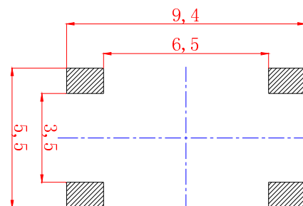
PCB参考图
