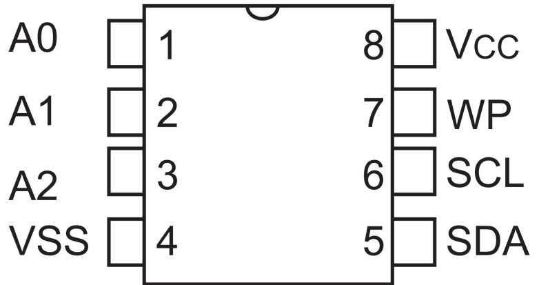
SOP8/DIP8/MSOP8
