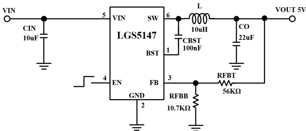
典型应用拓扑（VIN 大于 40V 时，须使用 10uH 及以上电感）
