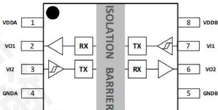
图 1.ADuM1286ARZ-HX/ADuM1286BRZ-HX SOP08(窄体)封装顶部视图
