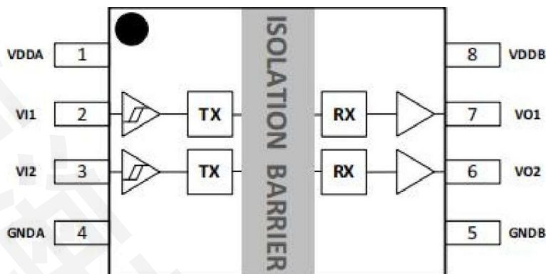
图 1.Si8423AB-D-IS-HX SOP08(窄体)封装顶部视
