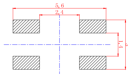
P C B 参考图
