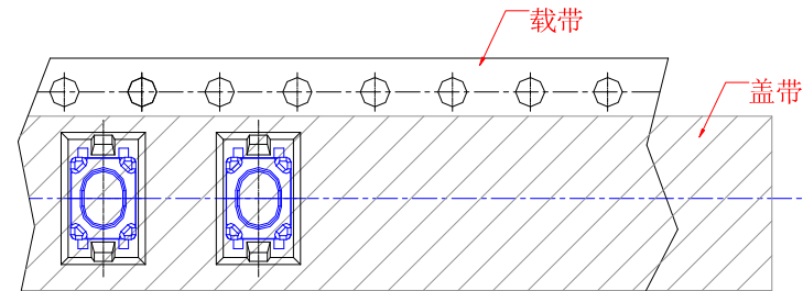
包装图
