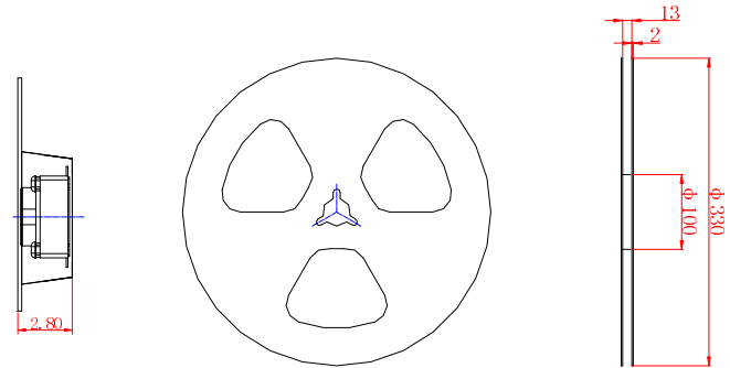
编带盘尺寸图
