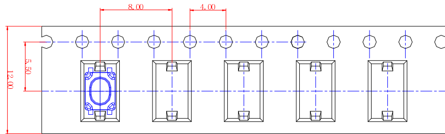
载带尺寸图
