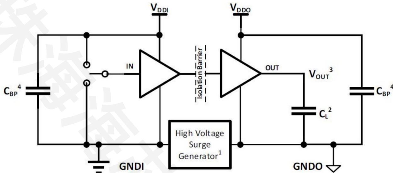
图 5. 共模瞬变抗扰度测试电路
