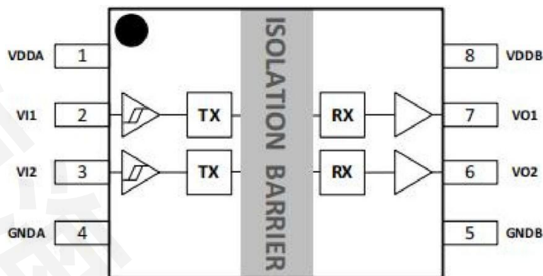
图 1.ISO7320FCDR-HX SOP-8(窄体)封装顶部视
