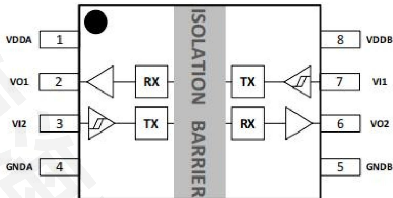
图 1.Si8426AB-D-IS-HX SOP08(窄体)封装顶部视图
