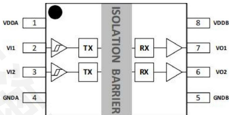
图 1.IS06720BDR-HX SOP08(窄体)封装顶部视
