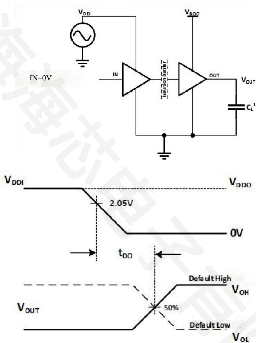
图 4. 默认输出延迟时间测试电路和电压波形
