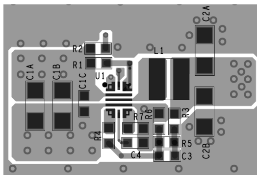
Top Layer
