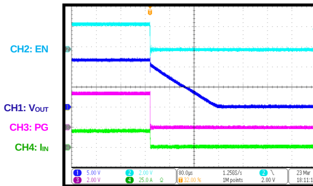
Shutdown via EN
