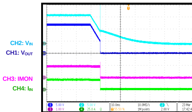
Shutdown via VIN
