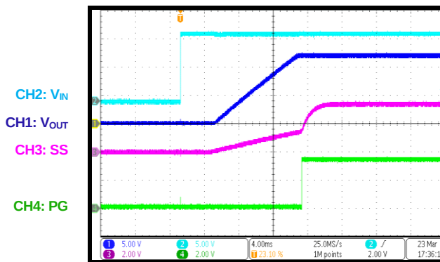
VIN Hot Plug
