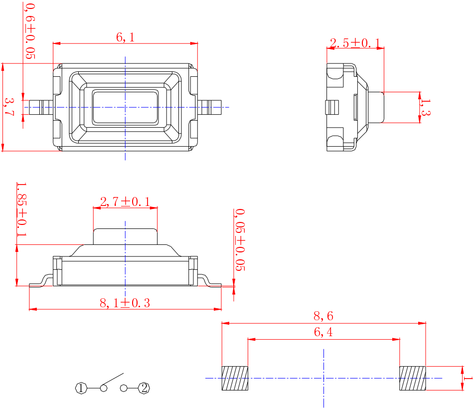
P C B 参考图
