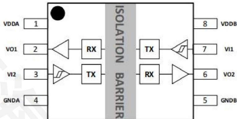
图 1.ISO6721FBDR-HX SOP08(窄体)封装顶部视图
