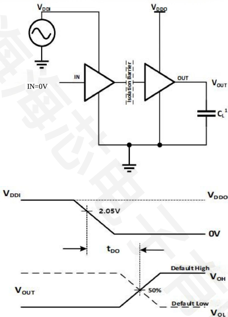
图 4. 默认输出延迟时间测试电路和电压波形
