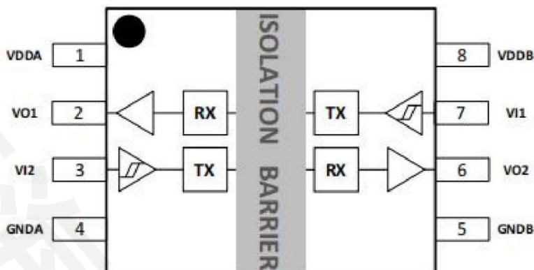
图 1. ISO7021DR-HX SOP08(窄体)封装顶部视图
