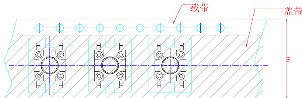
包装图
