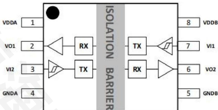
图 1. Si8422AB-D-IS-HXSOP08(窄体)封装顶部视图
