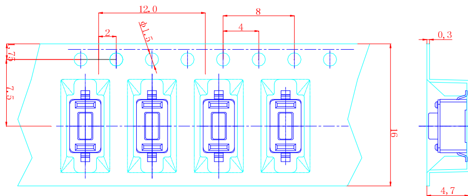
载带尺寸图
