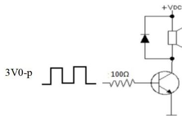
应用电路 application circuit
